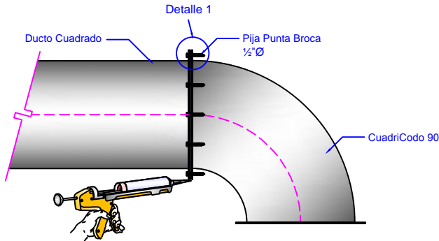
2. Montaje Lateral
