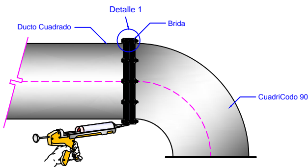
2. Montaje Lateral
