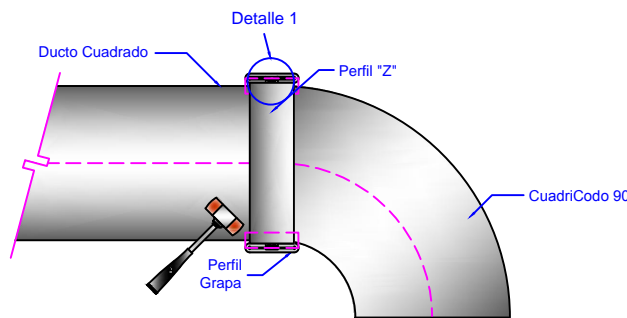
2. Montaje Lateral
